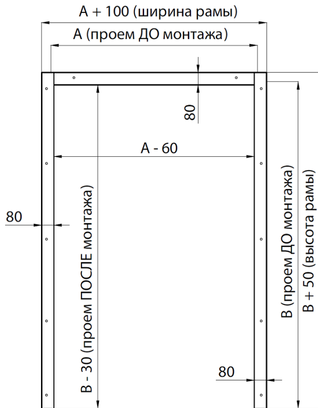
Рисунок 15. Металлическая рама «в обхват» проема
