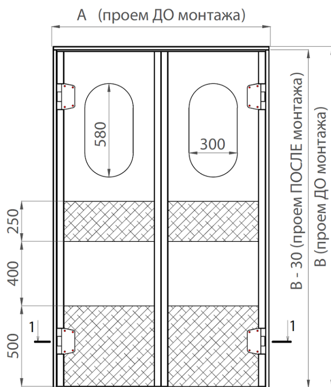
Рисунок 10. МДД с «П-образной» рамой
