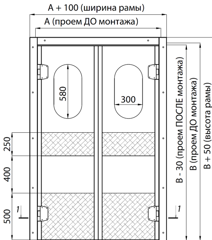
Рисунок 3. МДД с «угловой» рамой
