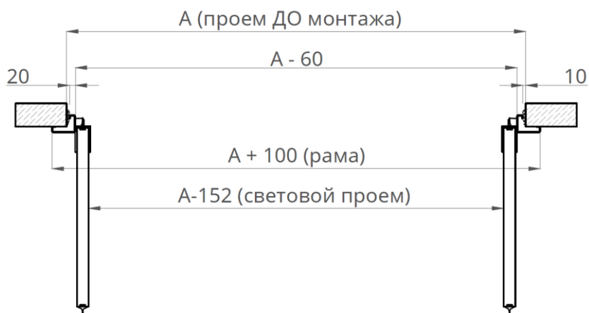
Рисунок 5. Разрез 1-1. МДД с плоским отбойником
