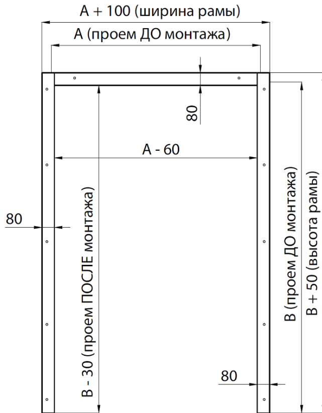
Рисунок 2. Металлическая «угловая» рама
