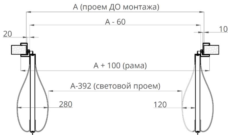
Рисунок 17. Разрез 1-1. МДД с изогнутым отбойником
