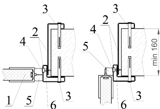
Рисунок 20: Узел 2. Крепление металлической рамы «в обхват» к кирпичной стене*
