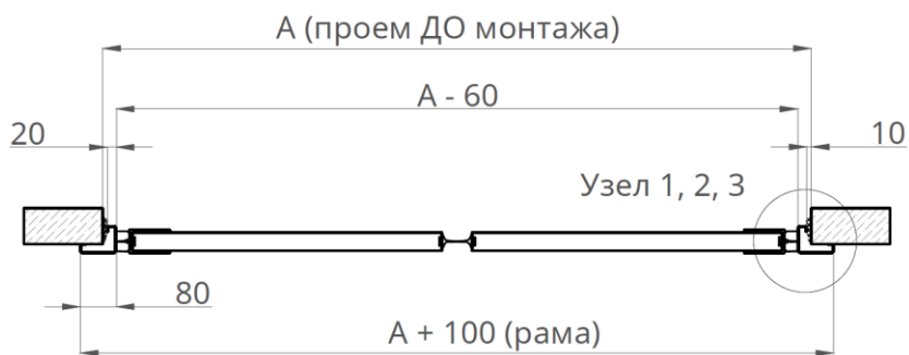
Рисунок 4. Разрез 1-1. МДД с изогнутым отбойником
