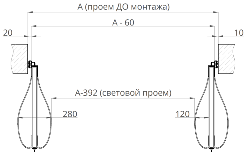
Рисунок 11. Разрез 1-1. МДД с изогнутым отбойником
