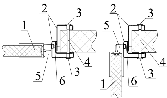
Рисунок 19: Узел 1. Крепление рамы «в обхват» к сэндвич-панели
