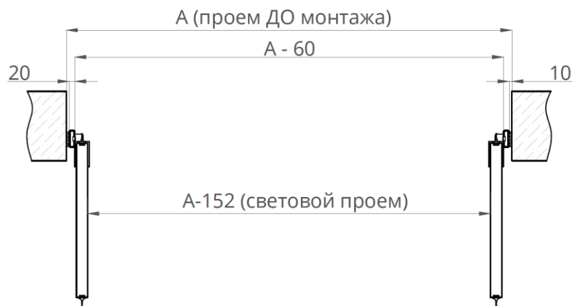
Рисунок 12. Разрез 1-1. МДД с плоским отбойником
