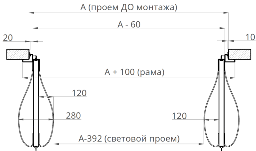
Рисунок 4. Разрез 1-1. МДД с изогнутым отбойником
