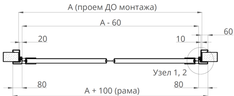
Рисунок 17. Разрез 1-1. МДД с изогнутым отбойником
