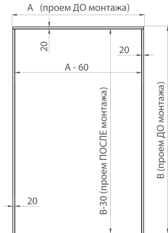
Рисунок 9. Металлическая «П-образная» рама
