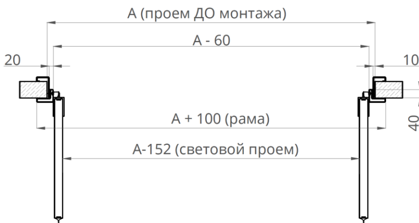
Рисунок 18. Разрез 1-1. МДД с плоским отбойником
