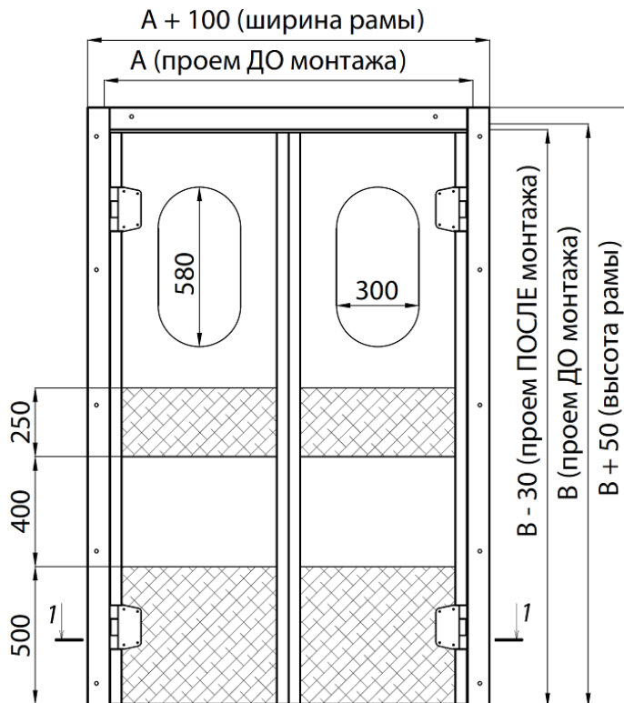
Рисунок 16. МДД с рамой «в обхват» проема
